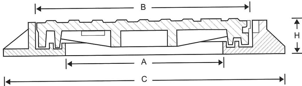
G.Y.牌18" 圓雙子口普通輕沙井(清水)
